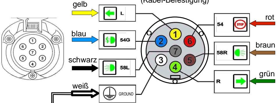
Anhängersteckdose 7-polig (Kabel-Befestigung)
